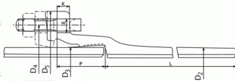
■接合部詳細圖 Detail drawing
